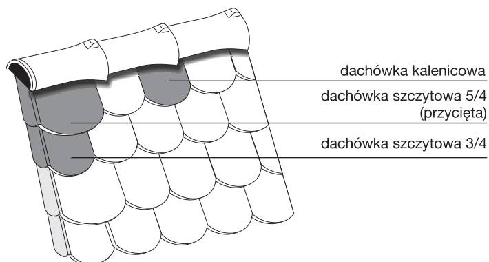
Rys. 24. Wykonanie kalenicy przy układzie w łuskę – zastosowanie dachówek kalenicowych
