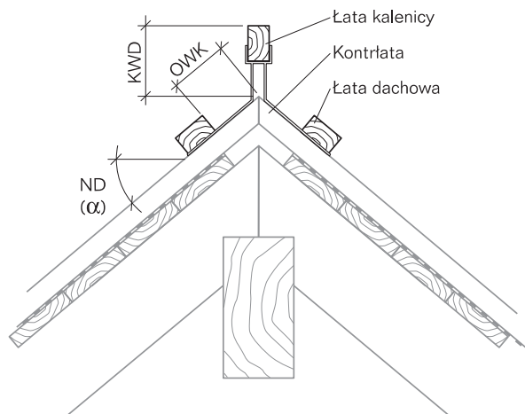
Rys. 23. Wymiary konstrukcyjne łąty kalenicowej
